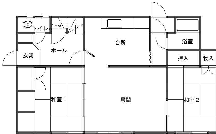
1階 間取り図 ※参考
